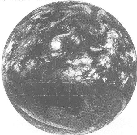
GMS-4 IR 0231 94 AUG 19 03Z
