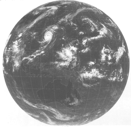
GMS-4 IR 0231 94 AUG 21 03Z
