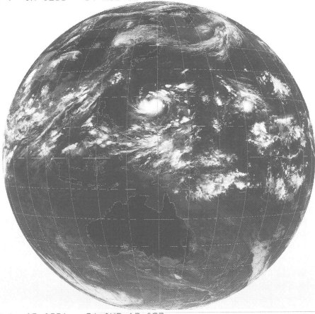
GMS-4 IR 0231 94 AUG 17 03Z
