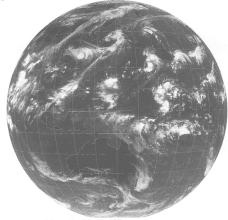
GMS-4 IR 0231 94 AUG 22 03Z
