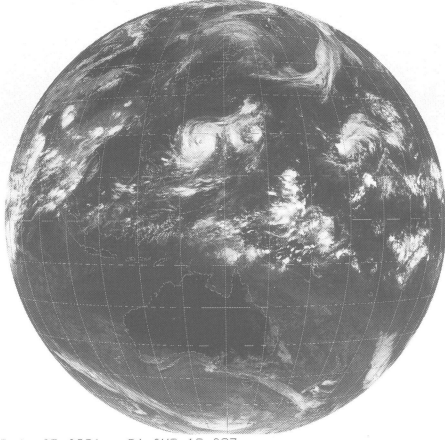
GMS-4 IR 0231 94 AUG 18 03Z
