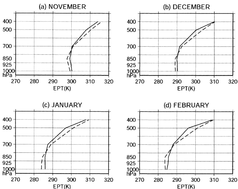
第6図 落雷日 (CG ≥ 1) と無落雷日 (CG = 0) のカテゴリー別の相当温位の高度分布。輪島における9時の高層データ。落雷日は実線、無落雷日は破線で示す。(a) は11月、(b) は12月、(c) は1月、(d) は2月を示す。
