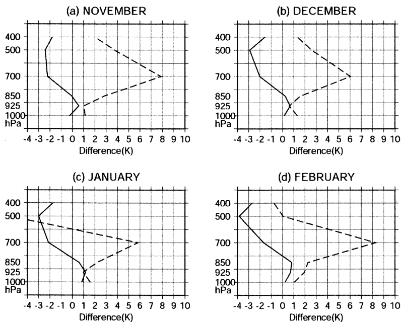
第7図 第6図と同様。ただし、落雷日と無落雷日との気温差(実線)と平均露点温度差(破線)の高度分布。
