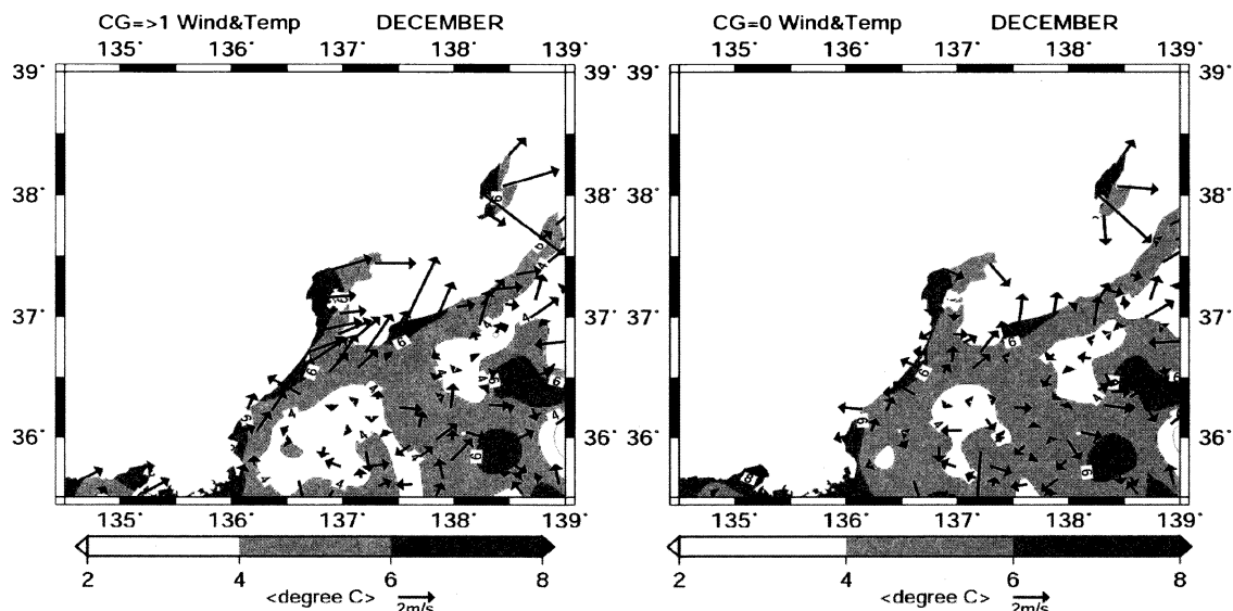
第9図 12月9時における落雷日(左)と無落雷日(右)の解析領域内のアメダス地上気温と風向風速。
