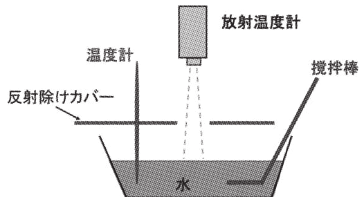
第5図 放射温度計の簡単な検定法。反射除けカバーは、放射で加熱(日中)または冷却(夜間)しても水面側に影響しないよう、熱伝導の悪い材質(ダンボールなど)でつくる。
