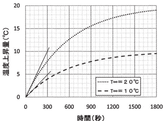
第4図 時定数が600秒の物体の温度上昇。点線は平衡状態のときの温度上昇が20 ^{\circ}\text{C} 、破線は10 ^{\circ}\text{C} の場合。
