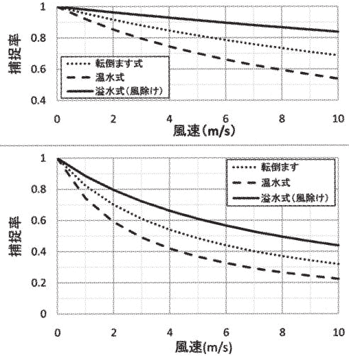
第6図 雨量計受水口付近の風速と降水粒子の捕捉率，上図：液体降水，下図：固体降水（中井・横山（2009）に基づき作図）。
