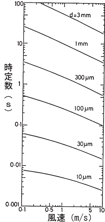
第2図 風向に垂直な円柱状温度センサーの時定数と風速の関係、パラメータは直径。ただしセンサーの体積熱容量 =4.2 \times 10^6 J/Km 3 のとき（近藤 1982）。
