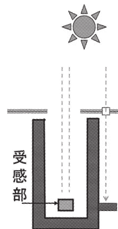
第3図 直達日射量を測る原理。受感部に短い円柱の銀を用いた銀盤日射計がある。
