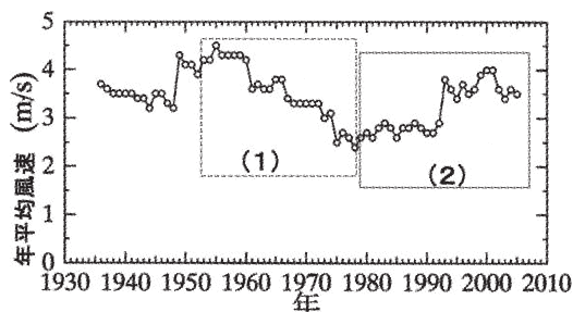
第1図 函館における1935年以降の70年間の年平均風速の経年変化。図中の(1)、(2)は本文を参照。
