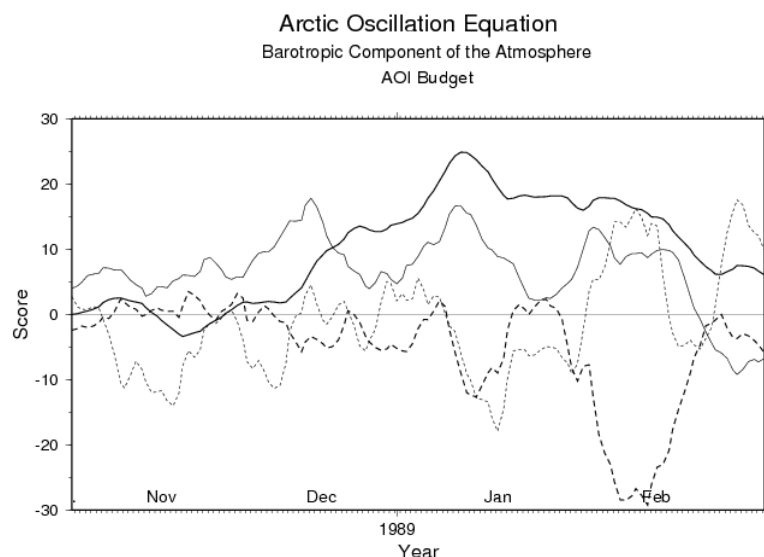
図 4 1988 年 11 月 から 1989 年 2 月の A0I と A0I 方程式各項の時系列 (本文参照)
