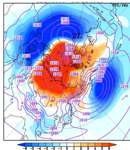
図1 2009/2010 年 DJF 平均 SLP アノマリの分布
