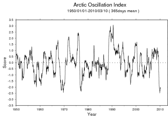
図 2 大気の順圧成分の EOF-1 による 1950-2010 年の AOI の時系列
