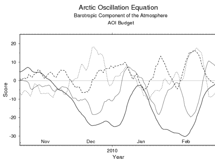
図 3 2009 年 11 月 から 2010 年 2 月の AOI と AOI 方程式各項の時系列 (本文参照)
