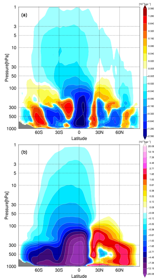
第 12 図 質量流線関数の BSISO phase5(振幅 2σ以上)の緯度-高度断面 3 日後ラグ合成図 (a)は平年偏差の合成図、(b)は実況図の合成図をそれぞれ表す。単位はいずれも 10^{10} \text{ kg s}^{-1} 。フィルターは施していない。
