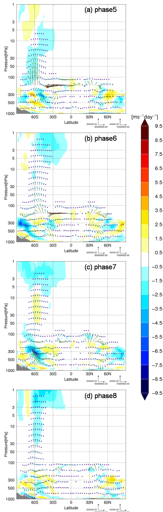
第9図 第8図と同様、ただし要素はEP flux 偏差(ベクトル)およびその収束・発散偏差(陰影)
