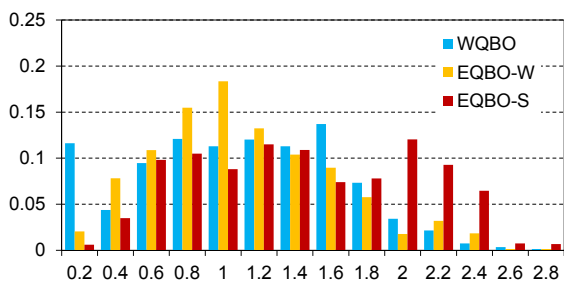
第 15 図 QBO-U20 の位相別にみた BSISO の振幅の規格化した出現頻度分布図
