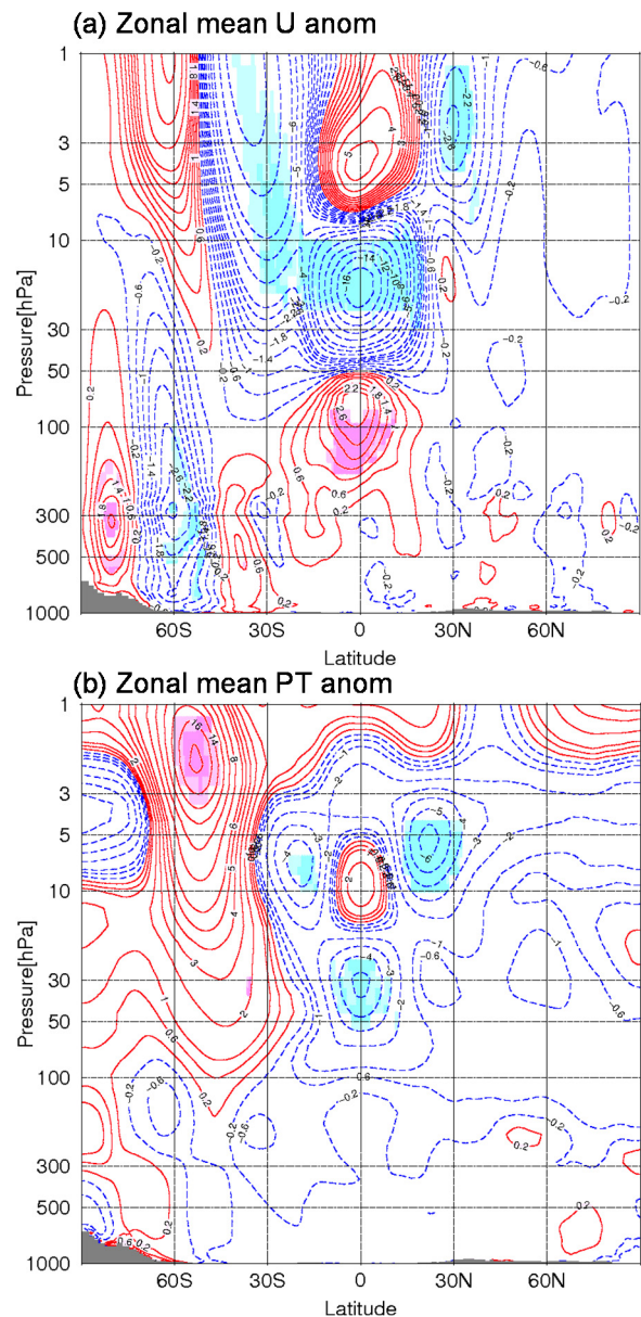
第 14 図 BSISO phase3(振幅 2σ以上)における東西風および温位偏差の緯度-高度断面同時合成図 (a)および(b)は、東西風偏差( m s^{-1} )、温位偏差(K)をそれぞれ表す。(a)の図中の濃い桃色(水色)陰影は信頼度 95%、薄い桃色(水色)陰影は信頼度 90%で統計的に有意なことを示す。各要素には 90 日のローパスフィルターを施している。
