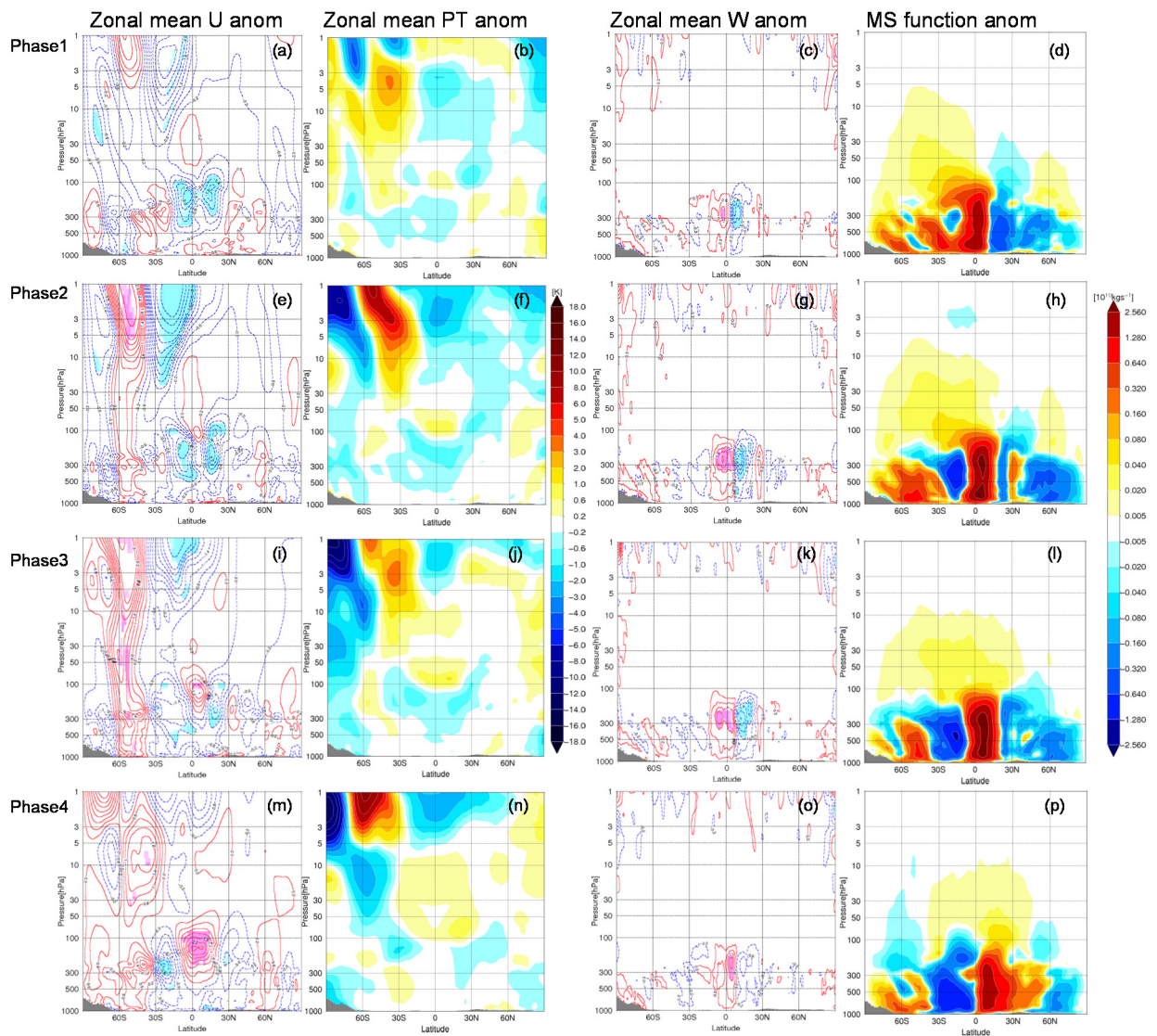
第 6 図 BSISO phase1~4(振幅 2 σ以上)における大気循環場各要素の平年偏差の緯度-高度断面同時合成図 左列から順に東西風偏差( \text{m s}^{-1} )、温位偏差(K)、鉛直流偏差( \text{m s}^{-1} )および質量流線関数偏差( 10^{10} \text{ kg s}^{-1} )をそれぞれ表す。東西風偏差図中の赤(青)線は、西(東)風偏差を、鉛直流偏差図中の赤(青)線は上昇流(下降流)をそれぞれ表す。また東西風偏差図、鉛直流偏差図中の濃い桃色(水色)陰影は信頼度 95%、薄い桃色(水色)陰影は信頼度 90%で統計的に有意なことを示す。各要素には 25~90 日のバンドパスフィルタを施している。
