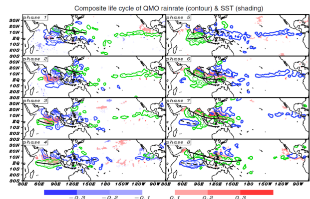
第 2 図 BSISO を 8phase に分けた降水量偏差と SST 偏差の合成図 (Wang et al.(2006)より引用)
