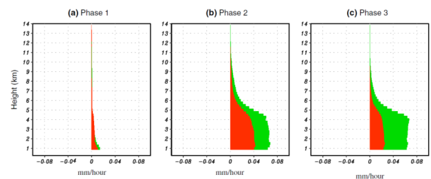
第 3 図 BSISO の Phase1~3 に対するインド洋赤道域(5°S-5°N、60°-70°E 平均)降水量偏差の鉛直分布の合成図 (Wang et al.(2006)より引用)
