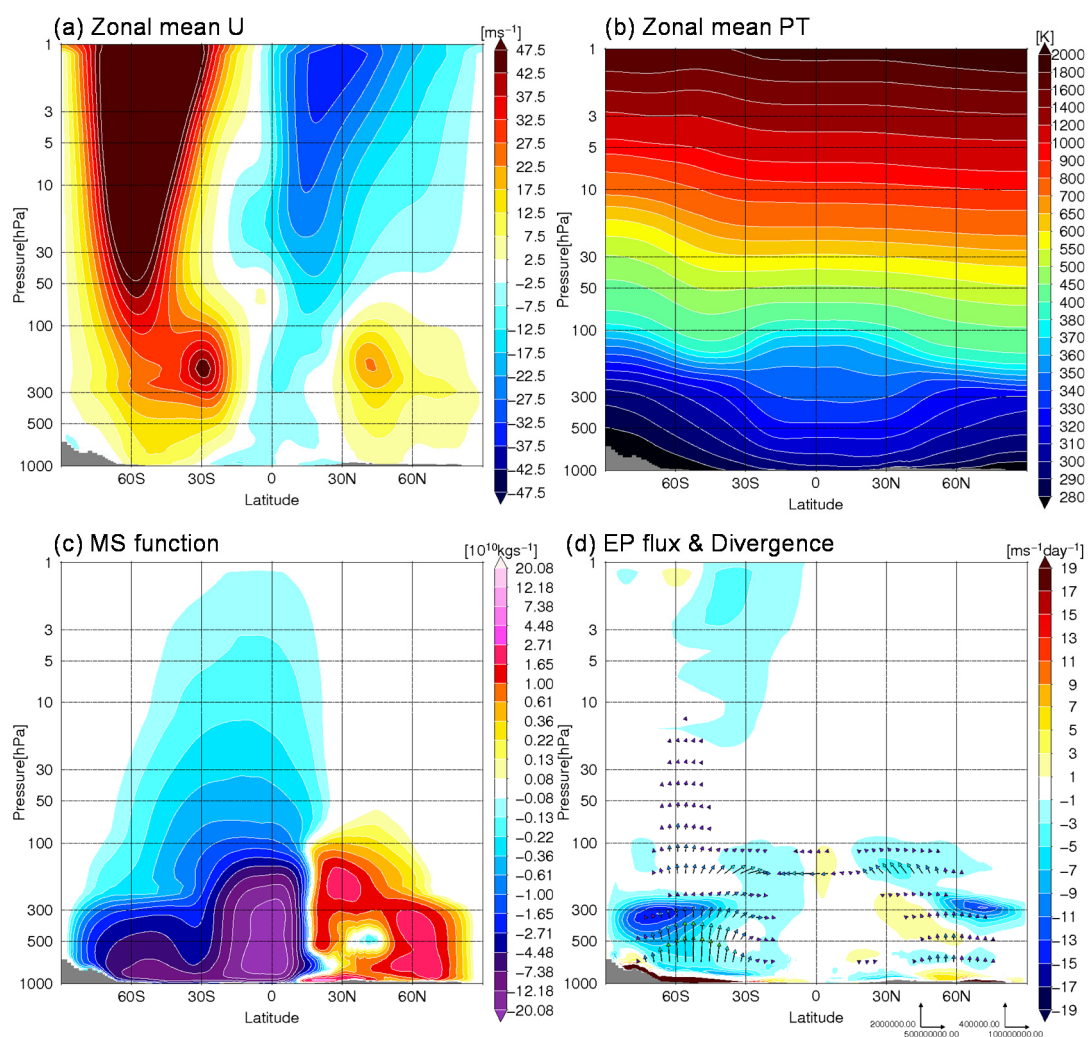
第 5 図 大気循環場各要素の北半球夏季(6~8 月平均) 平年値の緯度-高度断面図
