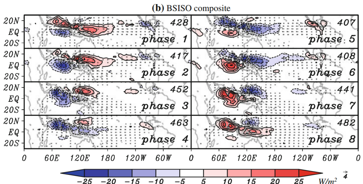
第 4 図 BSISO を 8 位相に分けた OLR 偏差(陰影)と 850hPa 風(ベクトル)の合成図(Kikuchi et al. 2012 より引用) 陰影域は OLR 偏差( W m^{-2} )を、ベクトルは 850hPa 気圧面における水平風( m s^{-1} )をそれぞれ表す。99%の信頼度でデータのみ描画。
