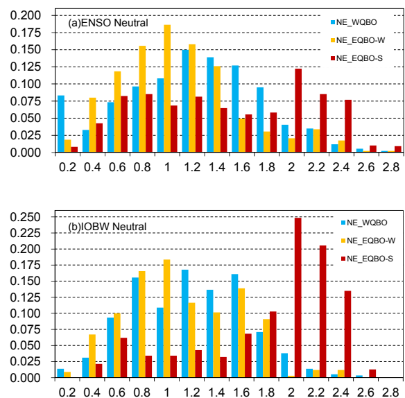
第 17 図 第 15 図と同様、ただし(a)ENSO ニュートラル時および(b)IOBW ニュートラル時において QBO-U20 の位相別にみた BSISO の振幅の規格化した出現頻度分布図
