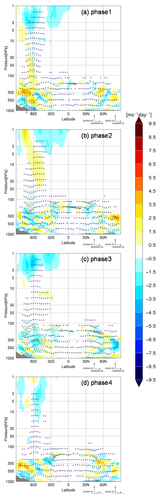
第7図 第6図と同様、ただし要素はEP flux 偏差(ベクトル)およびその収束・発散偏差(陰影)
