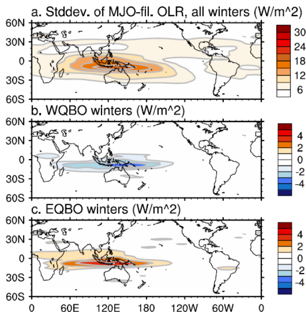
第 13 図 (a)冬季、波数 1-5、期間 20-100 日でフィルターされた OLR の標準偏差図、(b)QBO 西風位相時の(a)に対する偏差および(c)QBO 東風位相時の(a)に対する偏差(Yoo and Son(2016)より引用)
