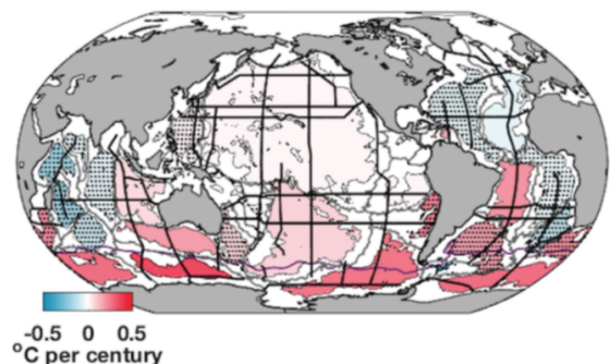
図 3 1981～2019 年の間で 4000m 以深における 100 年あたりの水温上昇率 (海洋・雪氷圏特別報告書 5 章 図 5.4)
