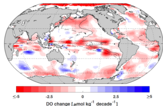
図 4 1960～2010 年の間で 1200m 以浅における 10 年あたりの O 2 の変化率(海洋・雪氷圏特別報告書 5 章 図 5.9)
