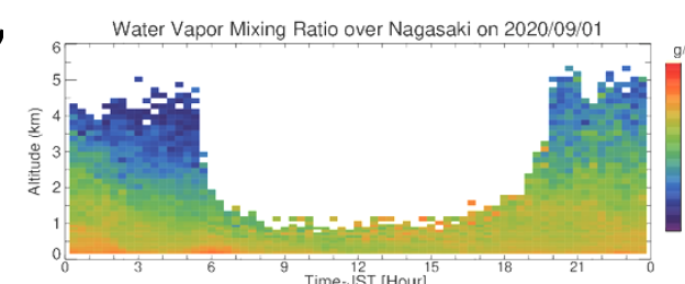
水蒸気観測
