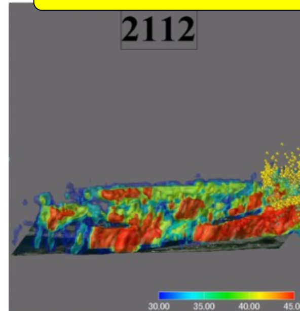
雷探知装置と気象レーダーによる三次元解析
