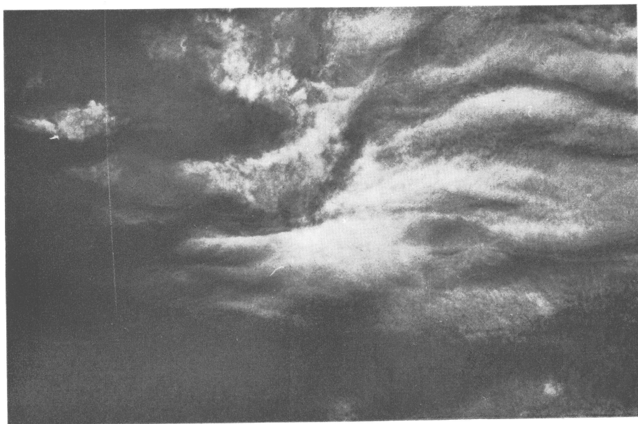
波状の巻積雲：層状をなした巻雲積で Cirrocumulus stratiformis undulatus すなわち巻積雲—層状—波状と分類される（筆者撮影）
