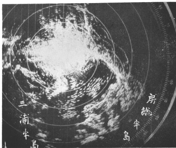
レーダーで捕えた東京湾内の船舶
