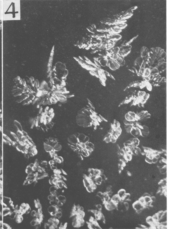
写真 同一のガラス面に成長した霜 (本文 212 頁参照)
