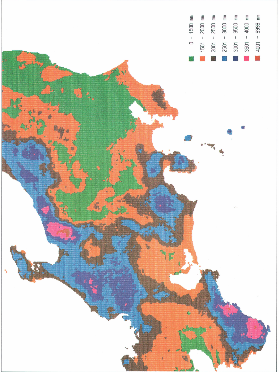
メッシュ年降水量分布図 (本文は157～174頁参照)
