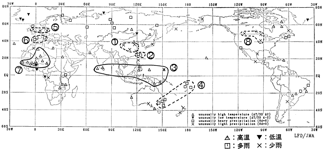
1988年4月の世界の異常天候分布図 図中の番号は、本文中の番号と対応している。
