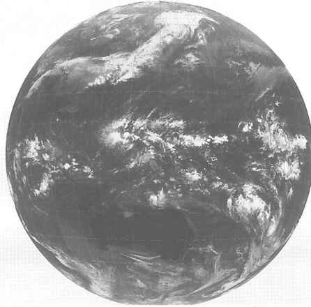
GMS-4 IR 0231 95 MAR 18 03Z
