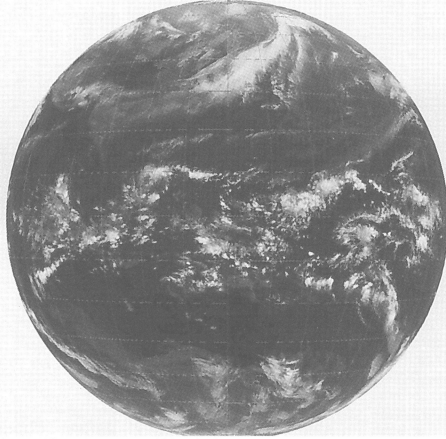
GMS-4 IR 0231 95 MAR 19 03Z
