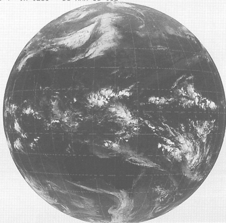
GMS-4 IR 0231 95 MAR 17 03Z
