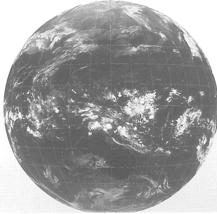
GMS-4 IR 2331 95 MAR 23 00Z
