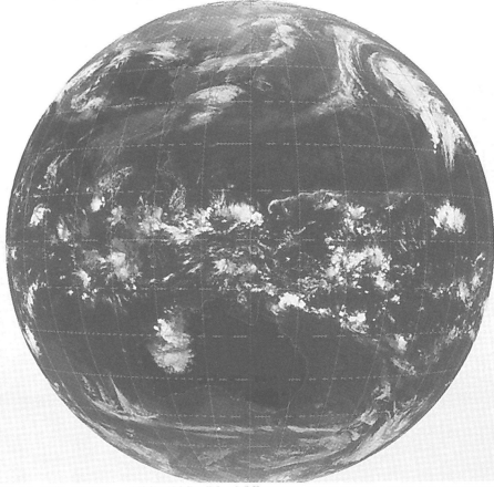
GMS-4 IR 0231 95 MAR 22 03Z
