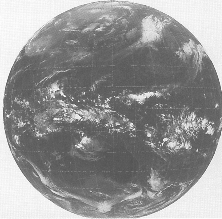
GMS-4 IR 0231 95 MAR 21 03Z
