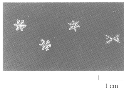
第1図 フォルムバール溶液で作成した天然の雪結晶のレプリカ。
