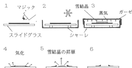
第2図 油性マーカーを使った vapour 法によるレプリカの作成手順。
