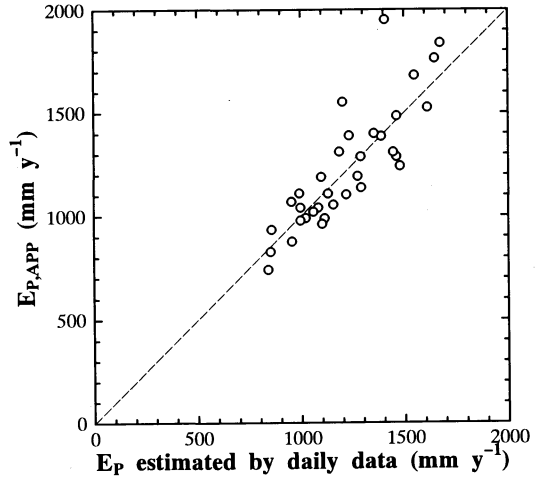
第3図 第2図と同じ、ただし縦軸は式(9)による小型蒸発計蒸発量と気温日較差の観測値から計算した年ポテンシャル蒸発量の推定値。
