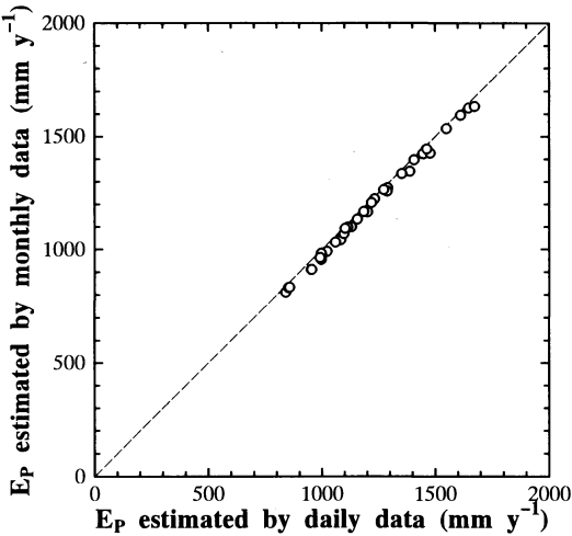
第2図 第1図と同じ、ただし年ポテンシャル蒸発量。
