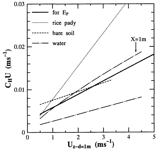
第4図 各種地表面の交換速度 C_H U と高度1mの風速 U_1 との関係。太い実線はポテンシャル蒸発量を生む仮想面、点線は粗な水田、広い水面は1点鎖線。 X=1m を付けた1点鎖線は大きさが1mの水面(近藤, 1994b, p.170)。破線は Matsushima and Kondo (1995) による裸地に対する関係。
