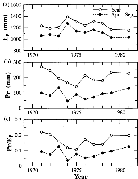
第5図 アルタイ (47.7N, 88.1E, 標高735 m) におけるポテンシャル蒸発量 (a), 降水量 (b), 気候湿潤度 (c) の年々変動。実線は年間値, 破線は4~9月の暖候期の値である。
