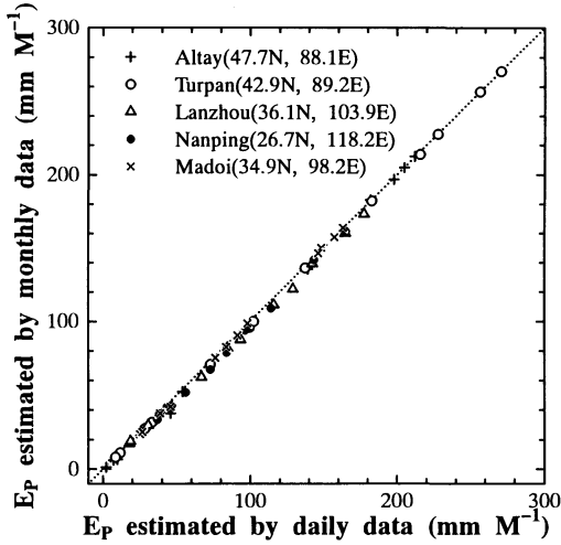
第1図 月ポテンシャル蒸発量の正確な計算値(横軸)と月平均気象要素を用いた近似計算値(縦軸)の比較。
