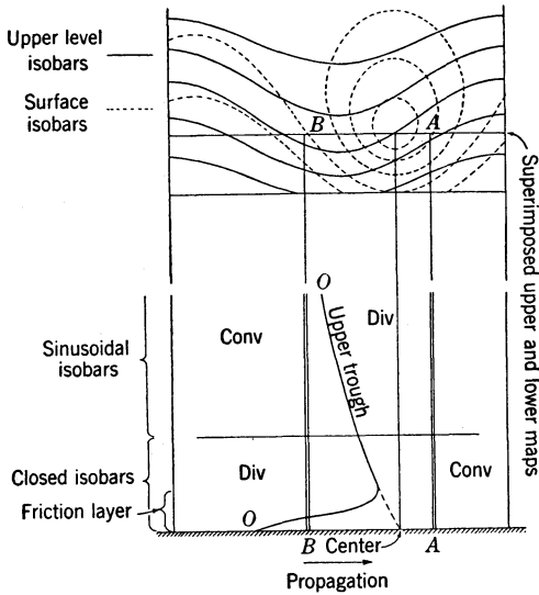
第1図 Bjerknnes and Holmboe (1944) による低気圧構造の模式図。上層下層の等圧線分布および収束発散，トラフ軸の西傾などが表現されている。
