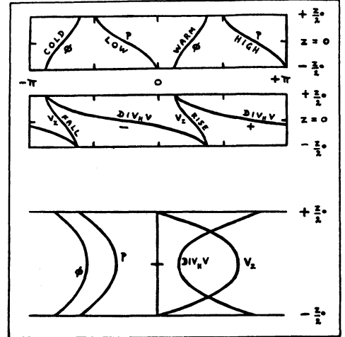
第2図 (上) Charney (1947) と(下) Eady (1949) の傾圧不安定理論による波の鉛直構造。第1図に対応する特徴が良く表現されている。
