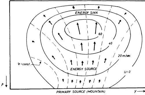
第4図 Eliassen and Palm (1961) によるロスビー波エネルギー伝播の概念図(子午面断面)。実線は平均東西風速, 矢印はエネルギーフラックスの向きと大きさを表す。
