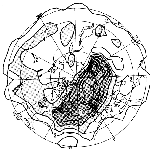
第3図 850 K の等温面（高度約30 km）における渦位 Q の分布図。1979年1月27日の例。（McIntyre and Palmer, 1983）。
