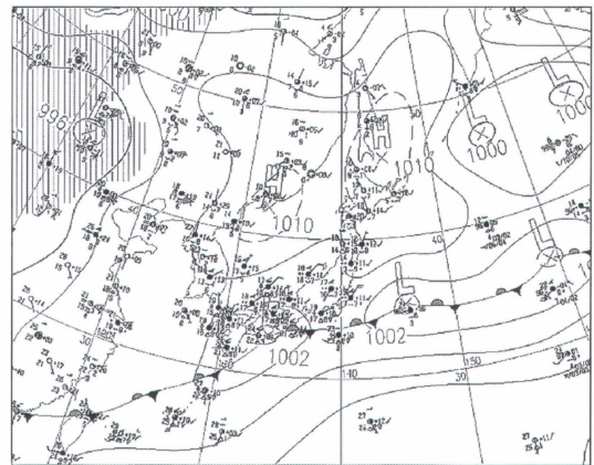
第 2 図 2001 年 (平成 13 年) 6 月 14 日 21 時地上天気図.
