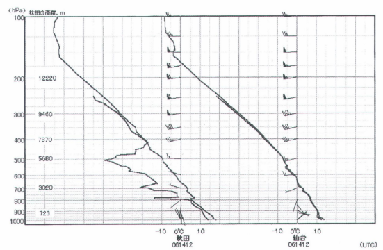
第 3 図 2001 年 (平成 13 年) 6 月 14 日 21 時秋田・仙台エマグラム. 縦軸は高度 (気圧, hPa), 横軸は温度 (°C), 秋田と仙台における気温 (右) と露点温度 (左) が示されている.
