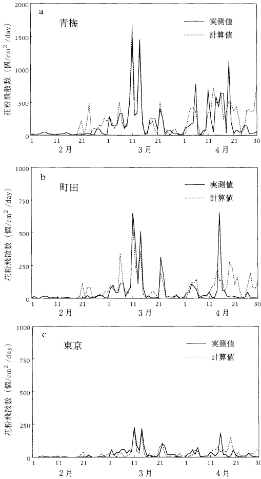
第7図 スギ花粉飛散数経時変化の実測値と計算値。 (a) 花粉の発生源に近い地点(青梅), (b) 花粉の発生源からすこし離れた地点(町田), (c) 花粉の発生源からかなり離れた地点(東京).
