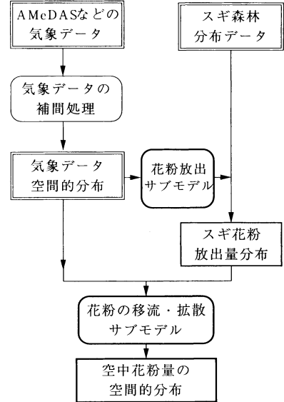
第5図 スギ花粉発生・拡散モデルの全体的構成。毎時気象データと、スギ森林の分布データをモデルに入力する。各気象要素の分布は、スギ花粉発生モデルおよび移流・拡散モデルへ入力する。
