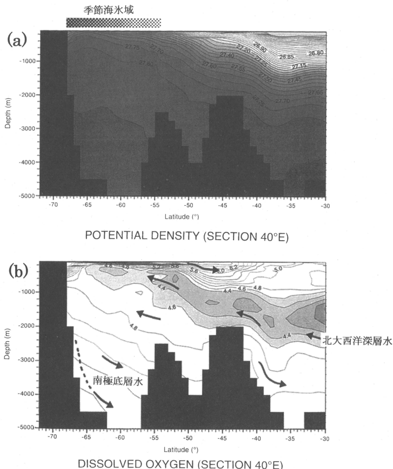
第1図 東経40度における、(a) ポテンシャル密度と、(b) 溶存酸素の子午面断面 (Olbers et al. , 1992より加筆)。
