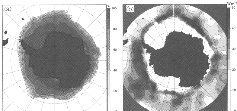
第3図 南大洋の8月における、(a) 平均海水密度度と、(b) 大気海洋(海水)間の正味の熱フラックスの標準偏差。ECMWF Re-Analysis ERA-15 (分解能 1.125^{\circ} ) のフラックスデータより計算(二橋創平氏作成)。
