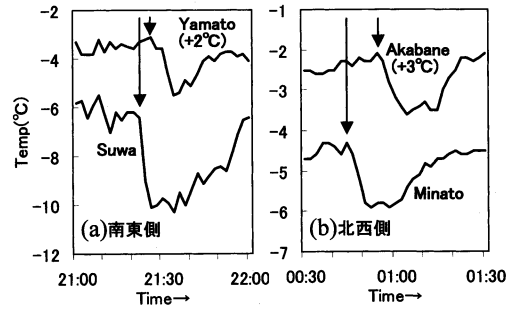
第9図 第8図について白抜き矢印で示した大きな気温低下の発生した時間帯を拡大した図。
