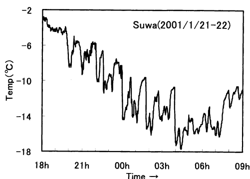
第2図 2001年1月21日18時から22日09時までの諏訪特別地域気象観測所の気温変化。
