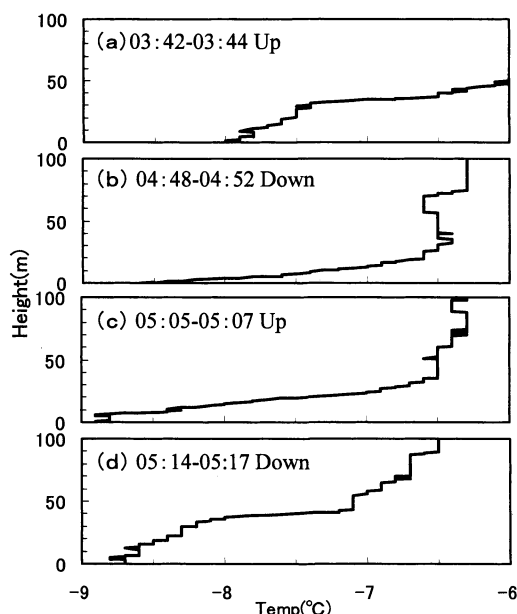
第11図 気温変動の発生した2003年1月26日の気温の鉛直プロファイル。観測時間はaが03時42～44分、bが04時48～52分、cが05時05～07分、dが05時14～17分。Upは係留気球の上昇時の観測、Downは下降時の観測を示す。
