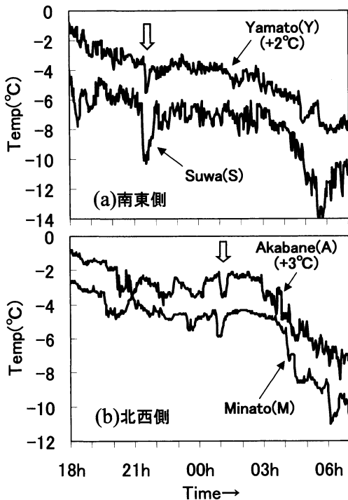
第8図 2003年1月25日18時～26日07時の気温経過。aは諏訪湖南東側の2地点(大和:Yamato, 諏訪特別地域気象観測所:Suwa), bは諏訪湖北西側の2地点(赤羽: Akabane, 湊: Minato)の気温経過。大和および赤羽は線が重ならないようにそれぞれ2°Cおよび3°Cプラス側にずらしている。
