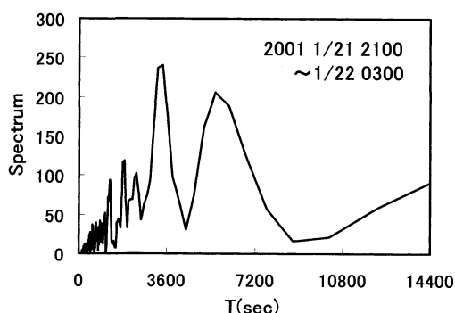
第3図 2001年1月21日21時～22日03時について、1次トレンドを除いてからFFT処理を行った結果。計算には1分間隔のデータを使用した。
