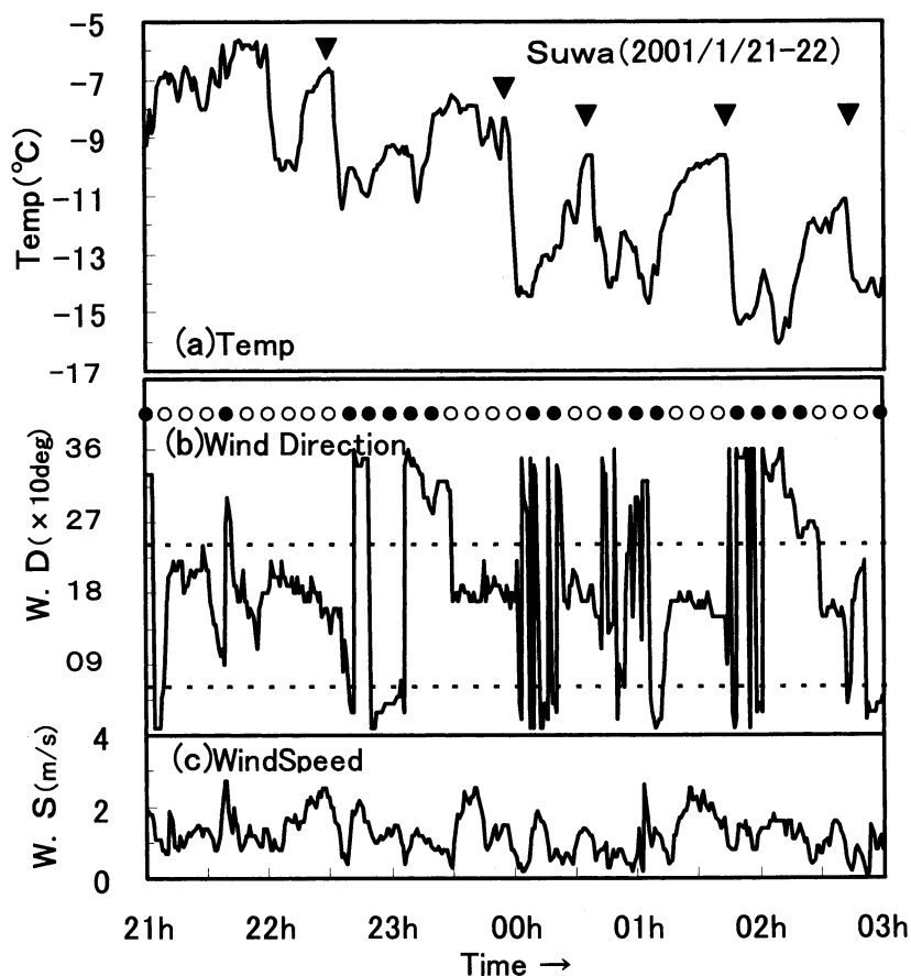
第4図 2001年1月21日21時～22日03時の諏訪特別地域気象観測所の観測値 (a:気温, b:風向, c:風速)。風向の破線は60°および240°, ○は風向が陸から, ●は風向が湖からであることを示す。
