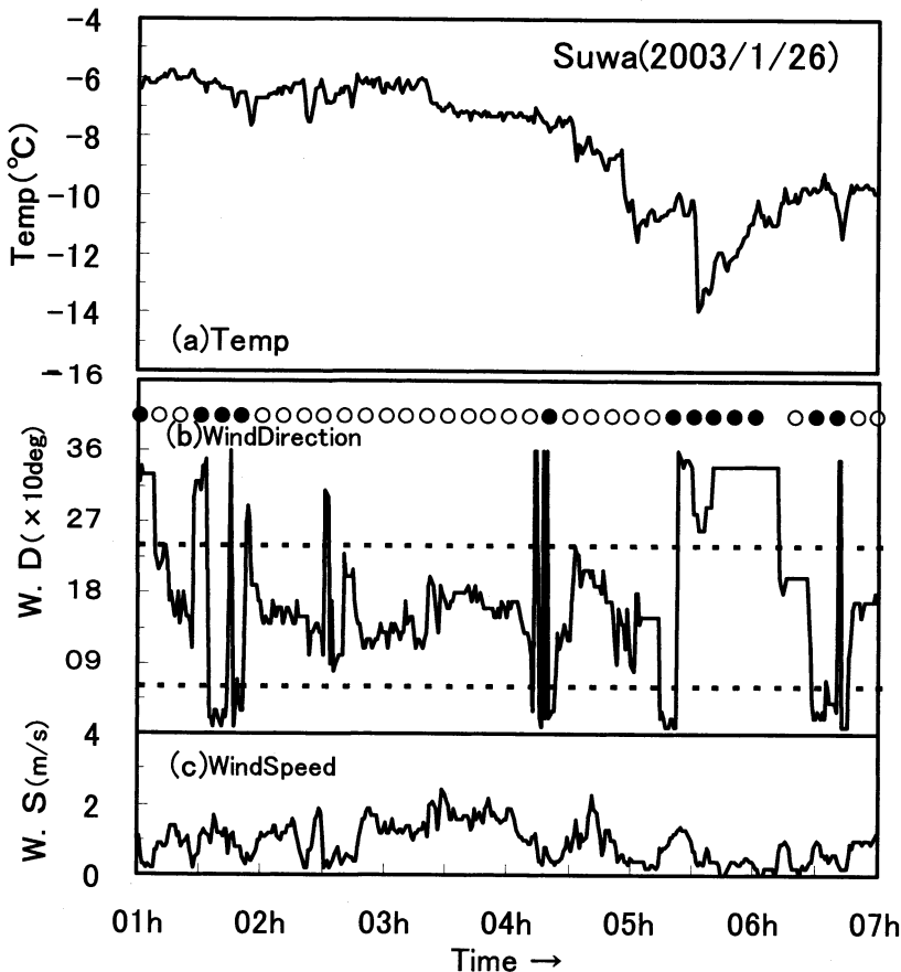
第6図 2003年1月26日01時～07時の諏訪特別地域気象観測所の観測値（a：気温，b：風向，c：風速）。記号は第4図と同じ。
