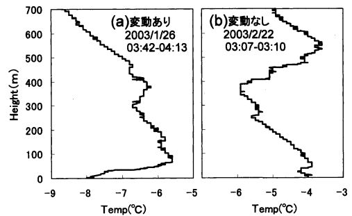
第10図 係留気球観測による気温の鉛直プロファイル (a: 気温変動の発生した2003年1月26日03時頃, b: 気温変動の発生していない2月22日03時頃)。
