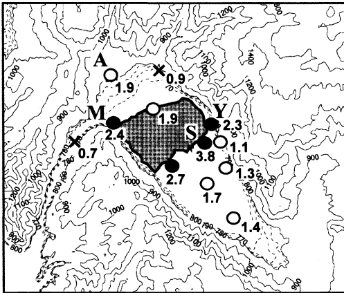
第7図 2003年1月25日18時～26日07時の気温変動幅(10分間気温差)の最大値。×は1°C未満, ○は1°C以上2°C未満, ●は2°C以上の地点。Y, S, A, Mは第8図で時系列を示す地点。
