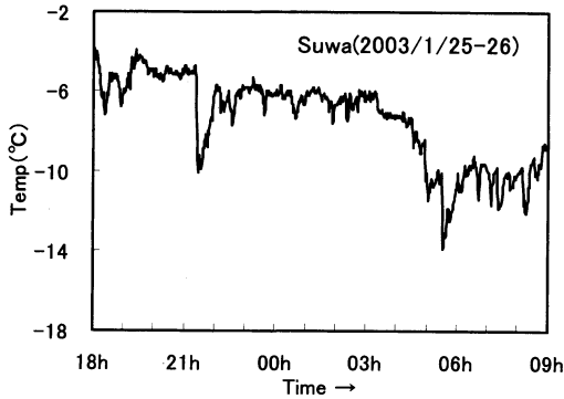
第5図 2003年1月25日18時から26日09時までの諏訪特別地域気象観測所の気温変化。
