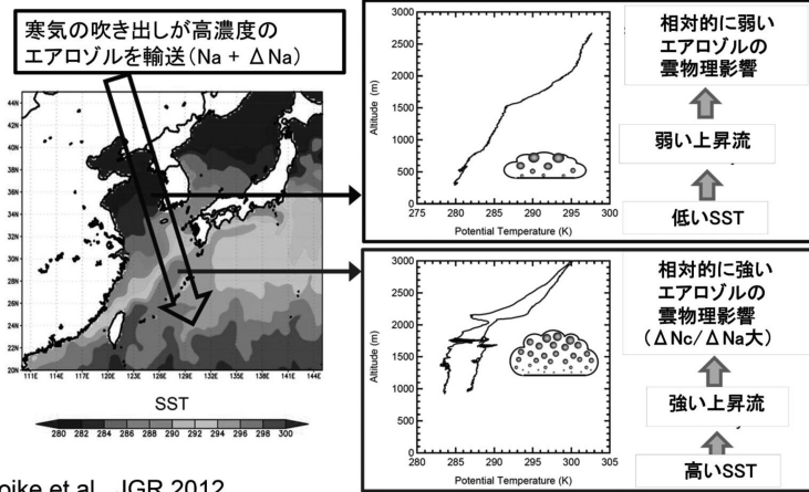
第1図 航空機観測から明らかとなった、大陸からの寒気の吹き出しに伴う雲粒子濃度の増大メカニズム (Koike et al. 2012).
